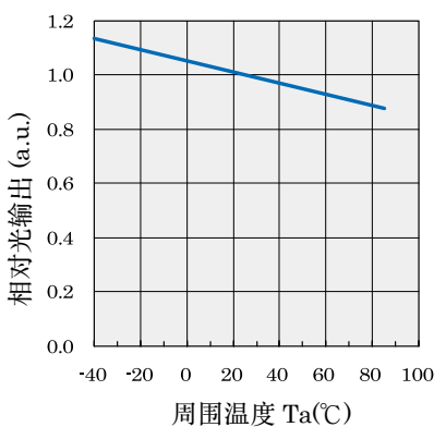
图 5. 相对光输出温度特性
