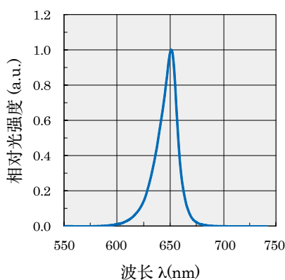
图 7. 发光光谱
