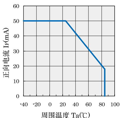
图 1. 降额曲线
