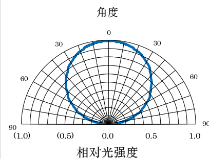
图 6. 指向特性
