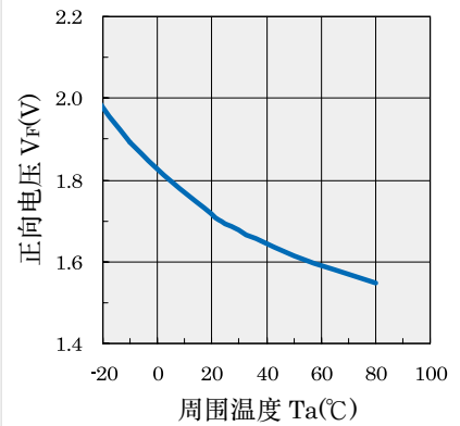
图 3. 正向电压温度特性
