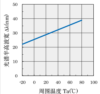
图 9. 光谱半值宽度温度特性
