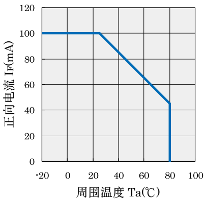
图 1. 降额曲线
