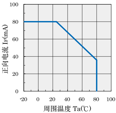
图 1. 降额曲线
