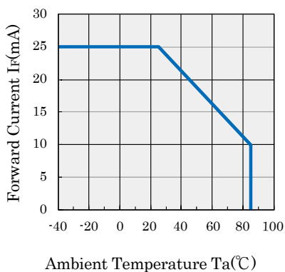
Fig1. I_F / T_a
