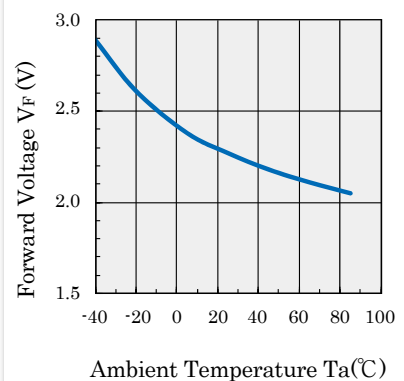
Fig3. V_F / T_a
